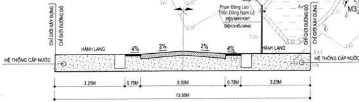
MẶT CẮT 1-1 ĐƯỜNG QH 13.5M
